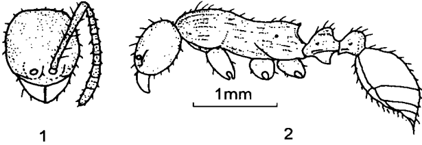
图 1~2 博白双节行军蚁新种 Aenictus bobaiensis sp. nov. 1. 头部正面观 head in frontal view; 2. 体侧面观 body in profile view.
