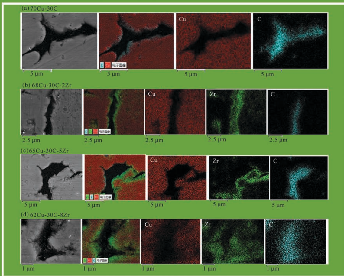
4种不同Zr体积含量的铜-石墨复合材料SEM-EDS图 (图片由本期作者张坤提供)
