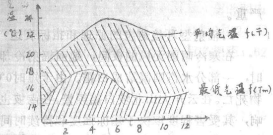
图1 南坡水平距离为山高倍数气温变化图
